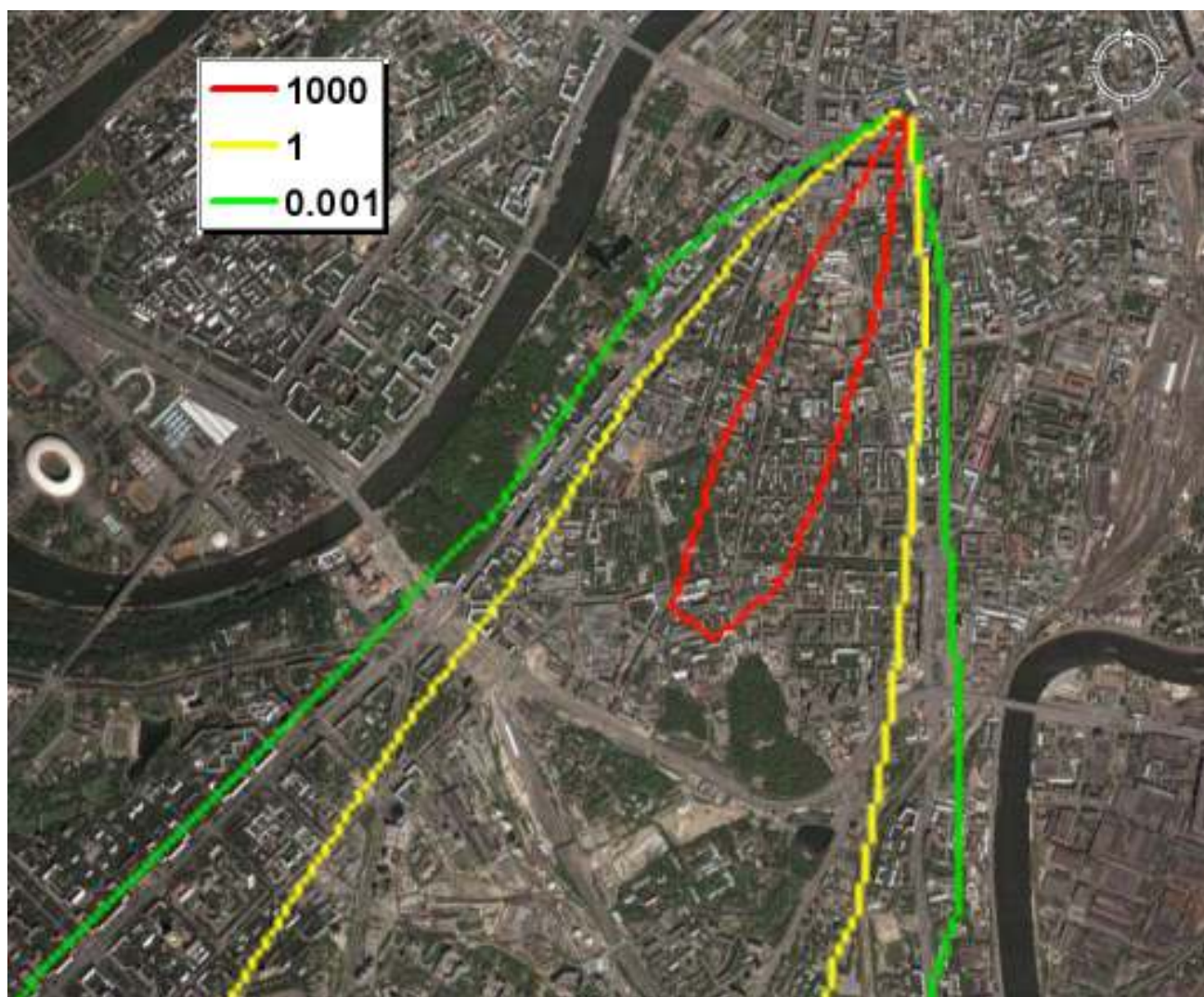
Рис. 4. Прогнозируемая плотность загрязнения местности на территории мегаполиса в случае диспергирования некоторого количества 137 Cs, Ки/км 2
