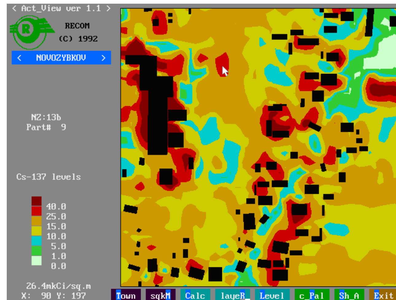
Рис. 5. Пример неравномерности радиоактивного загрязнения городской территории (Новозыбков, Брянская область, Российская Федерация)
